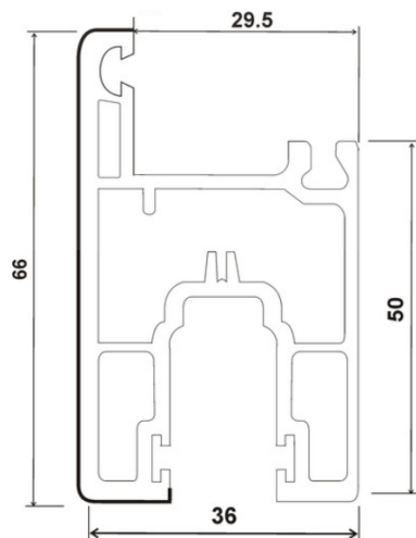
SP-80-MRS(B), SASH MONORAIL SLIDING (36*66)
