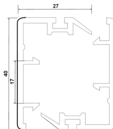
SP-80-IL , INTERLOCK WINDOW (27*40)
