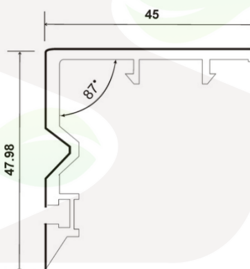
SP-DIL, INTERLOCK DOOR (45*48)
