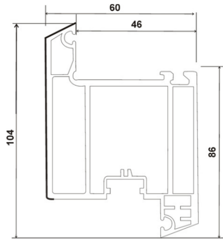
SP-60-CDS(I) , SASH CASEMENT INWARD DOOR (60*104)
