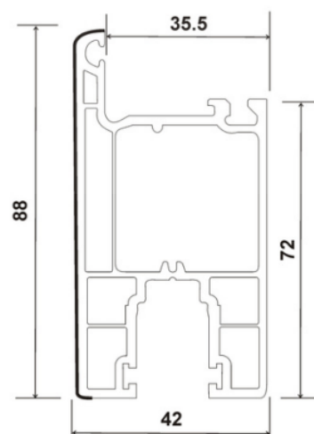
SP-DS , SLIDING DOOR SASH (42*88)
