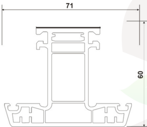
SP-60-ZT , MULLION T CASEMENT (60*71)
